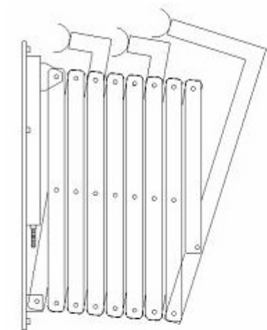
Zijaanzicht schaararm gesloten
